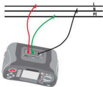
Рис. 22 Чередование фаз – подключение тестовых проводов
