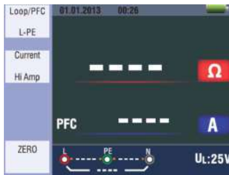
Рис. 6 Ожидание измерения в режиме Hi Amp
