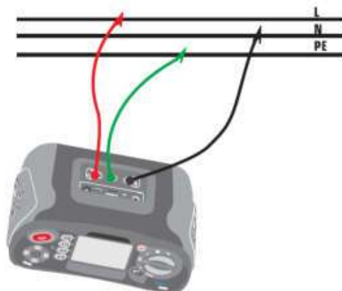
Рис. 12 Подключение тестовых проводов в режиме измерения сопротивления L-N
