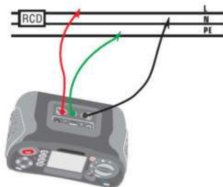
Рис. 15 Тестирование УЗО – подключение тестовых проводов
