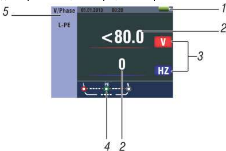
Рис. 1 Дисплей тестера
