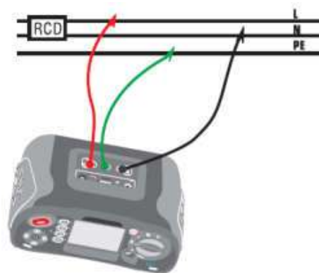
Рис. 4 Подключение тестовых проводов в режиме No Trip LOOP
