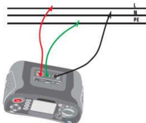
Рис. 8 Подключение тестовых проводов в режиме измерения Hi Amp LOOP
